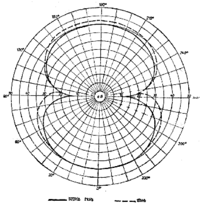
Směrová charakteristika
