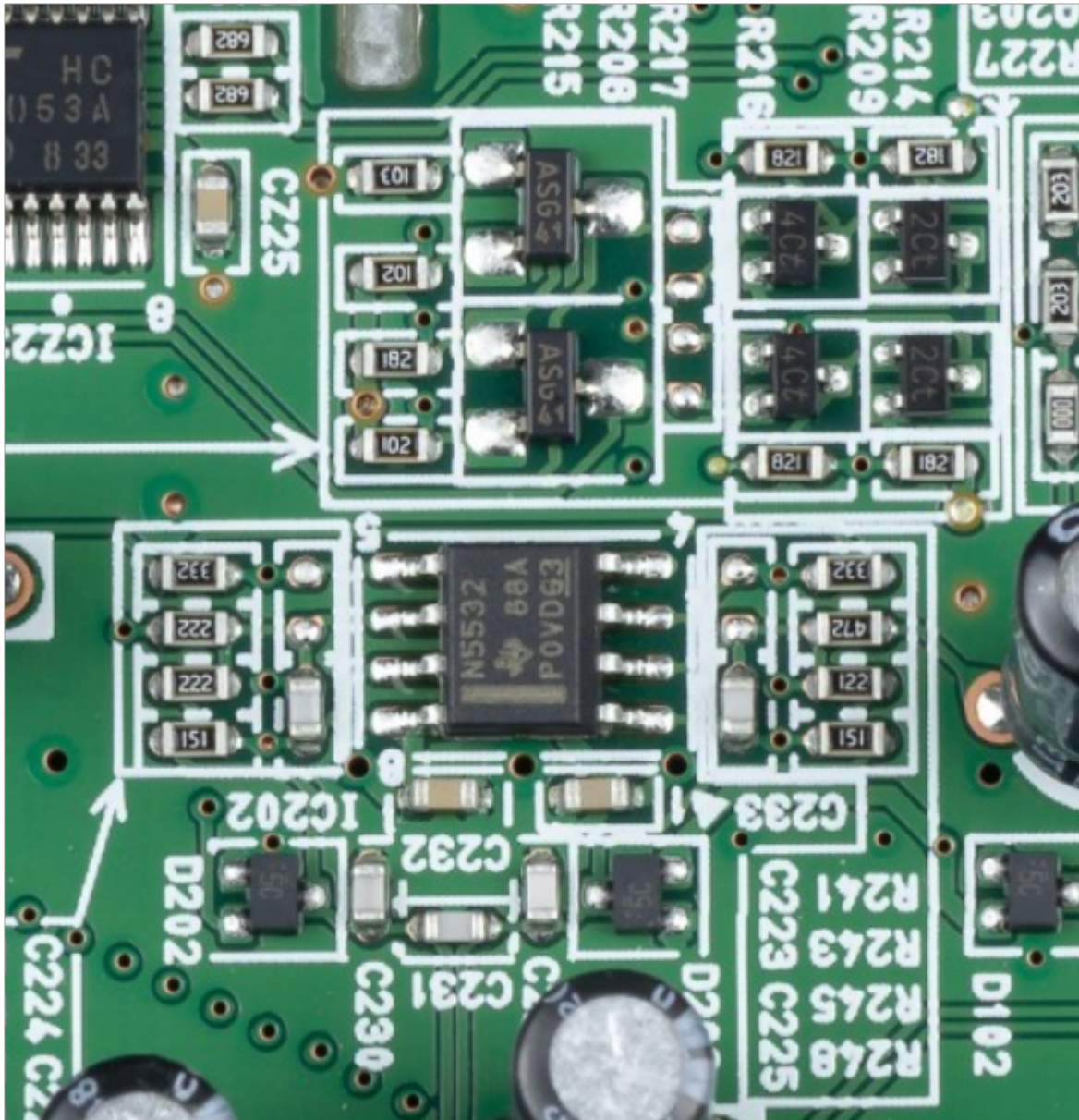
4 SMD NE5532 Op-Amp
