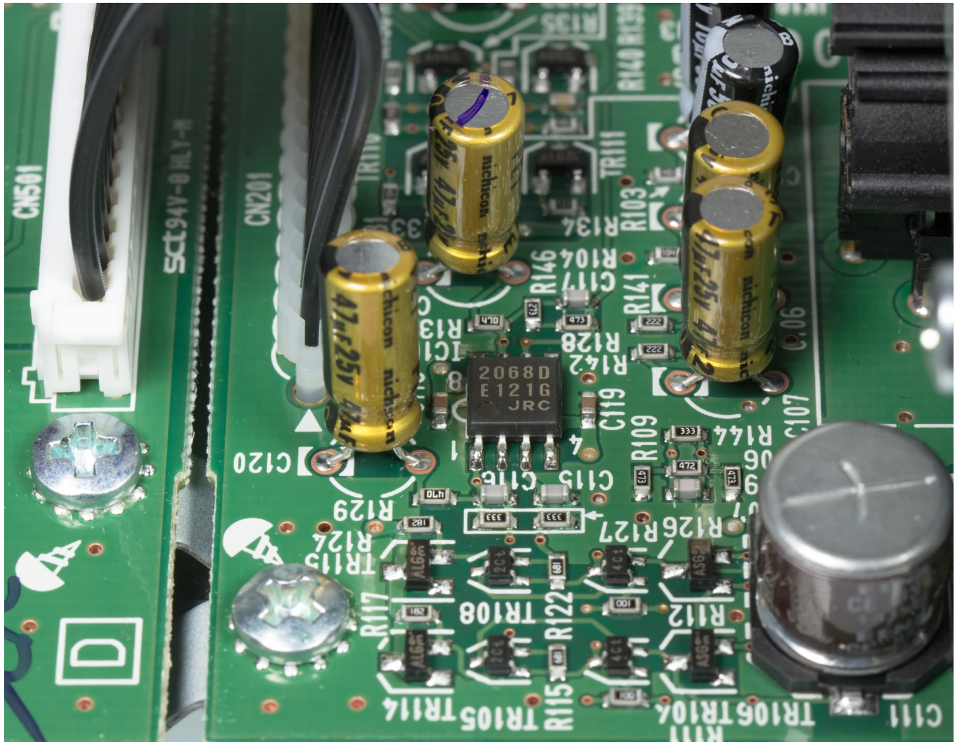
4 SMD JRC Op-Amp
